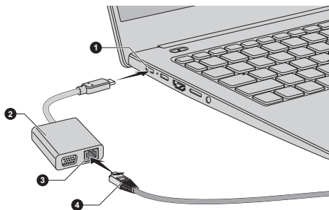
Rysunek 4-12 Podłączanie przewodu sieci LAN
