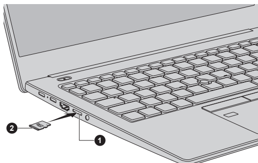
Rysunek 4-6 Instalowanie karty pamięci
