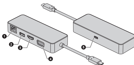
Rysunek 4-9 Adapter podrzędny USB-C™/HDMI™/VGA
