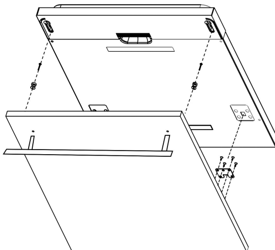
Rysunek 4a Instalacja panelu zabudowy drzwi.
