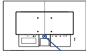
Dołączona śruba
