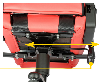
EN: Rocking function enable / disable in horizontal seat position PL: Opcja bujania z blokadą przy poziomej pozycji siedziska
