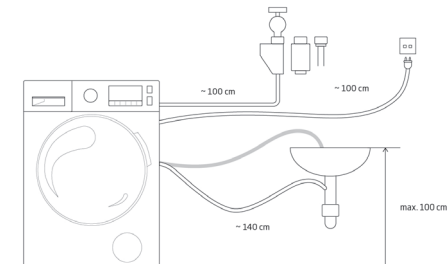
Przyłącze prawostronne
