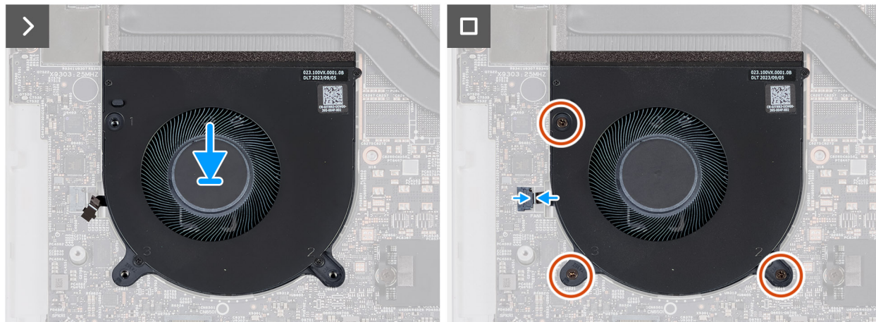
Rysunek 23. Instalowanie wentylatora karty graficznej
