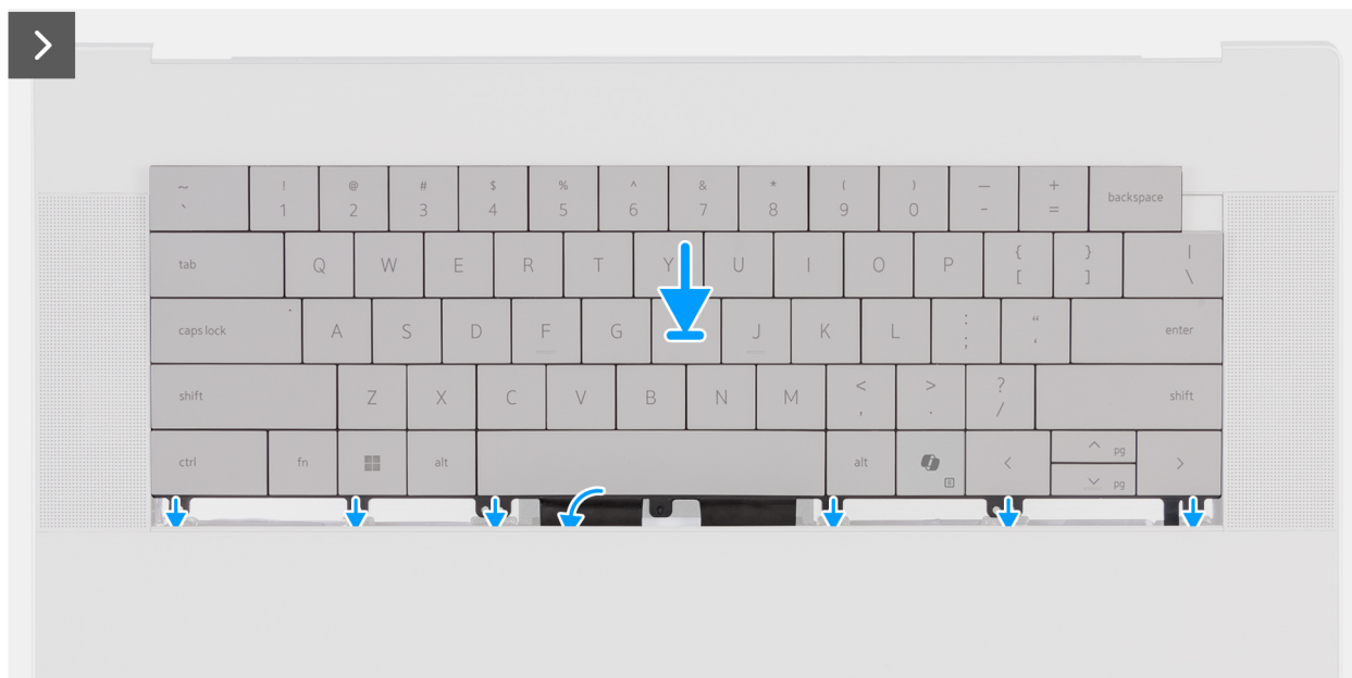
Rysunek 56. Instalowanie klawiatury
