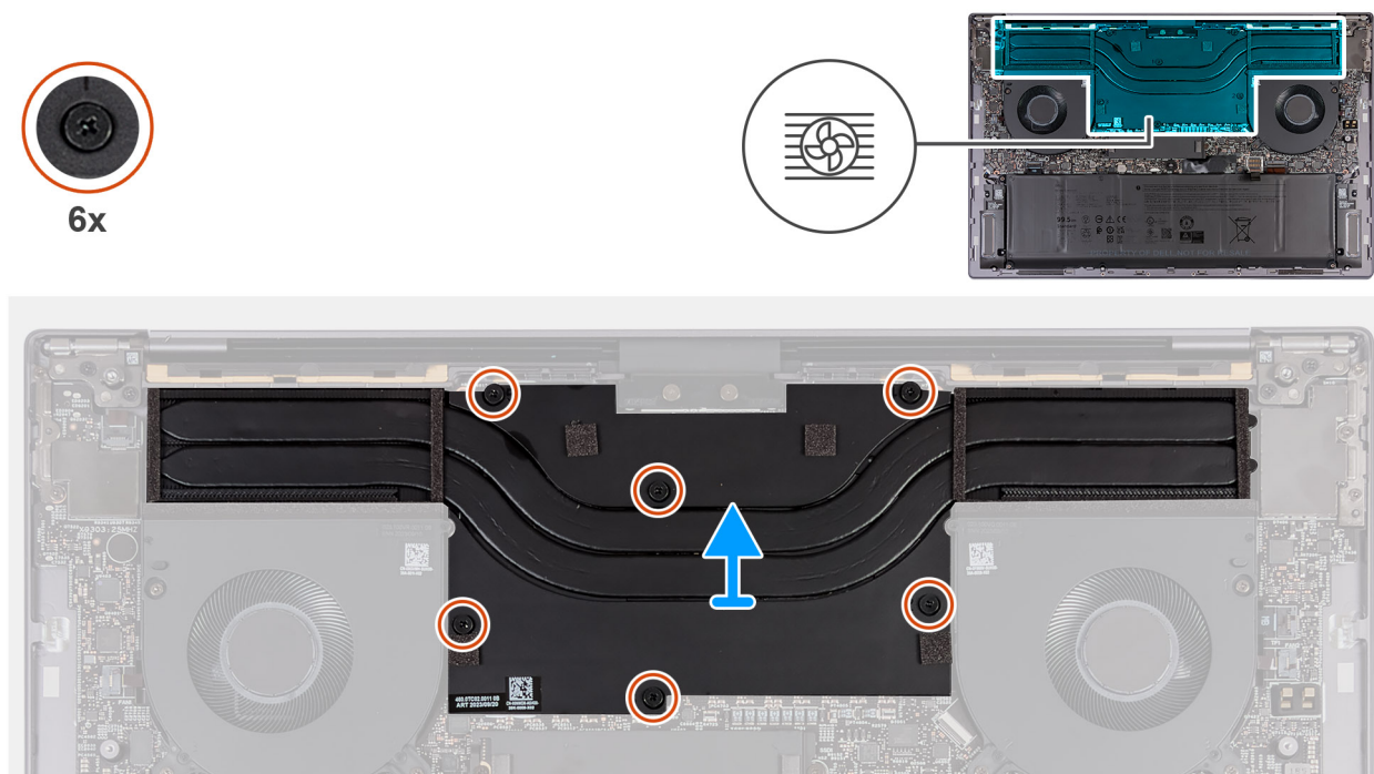
Rysunek 32. Wymontowywanie radiatora — konfiguracja z autonomiczną kartą graficzną (bez komory parowej)
