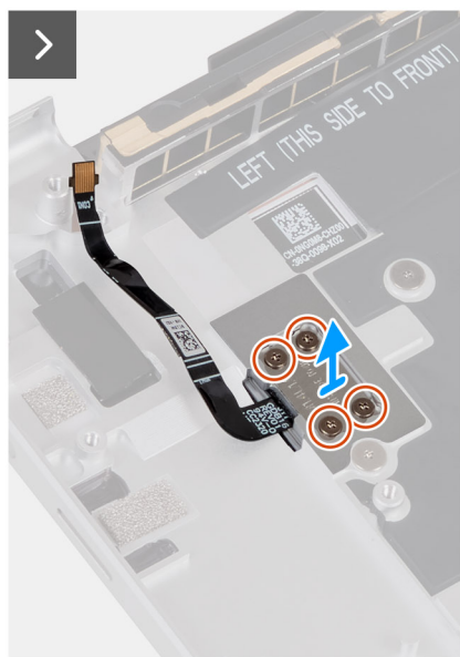
Rysunek 59. Wymontowywanie przycisku zasilania z czytnikiem linii papilarnych
