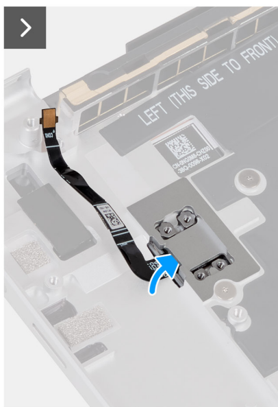
Rysunek 59. Wymontowywanie przycisku zasilania z czytnikiem linii papilarnych
