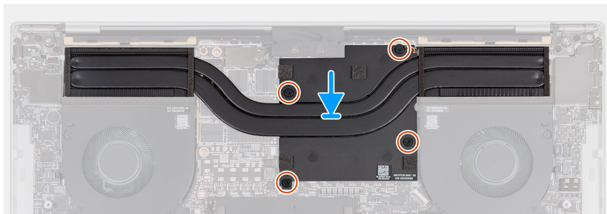
Rysunek 31. Instalowanie radiatora — konfiguracja ze zintegrowaną kartą graficzną
