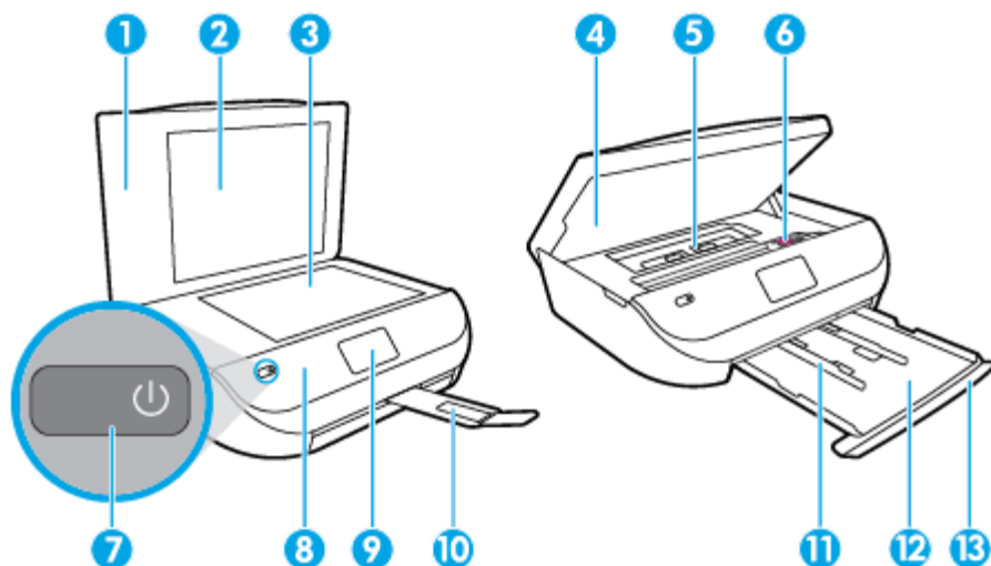
Rysunek 2-1 Widok urządzenia HP DeskJet Ink Advantage 4530 All-in-One series z przodu i z góry
