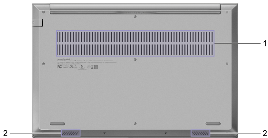
Rysunek 4. Widok z dołu—modele 15-calowe
